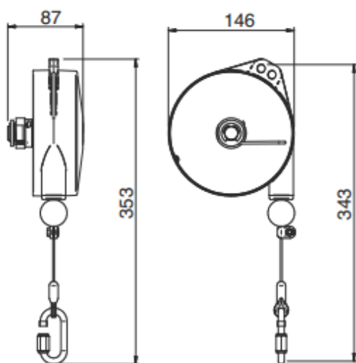
Plano dimensional serie X-light
