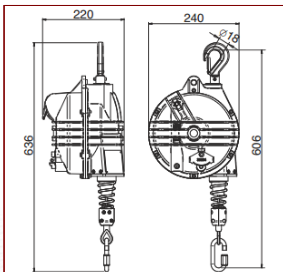
Plano dimensional serie Heavy
