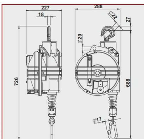
Plano dimensional 9401-9405 / 9431-9433
