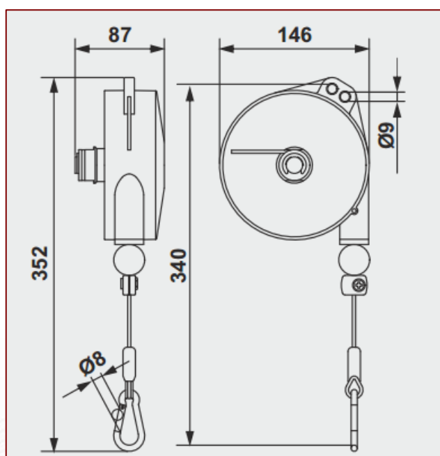
Plano dimensional 9320-9323 / 9320NY-9323NY
